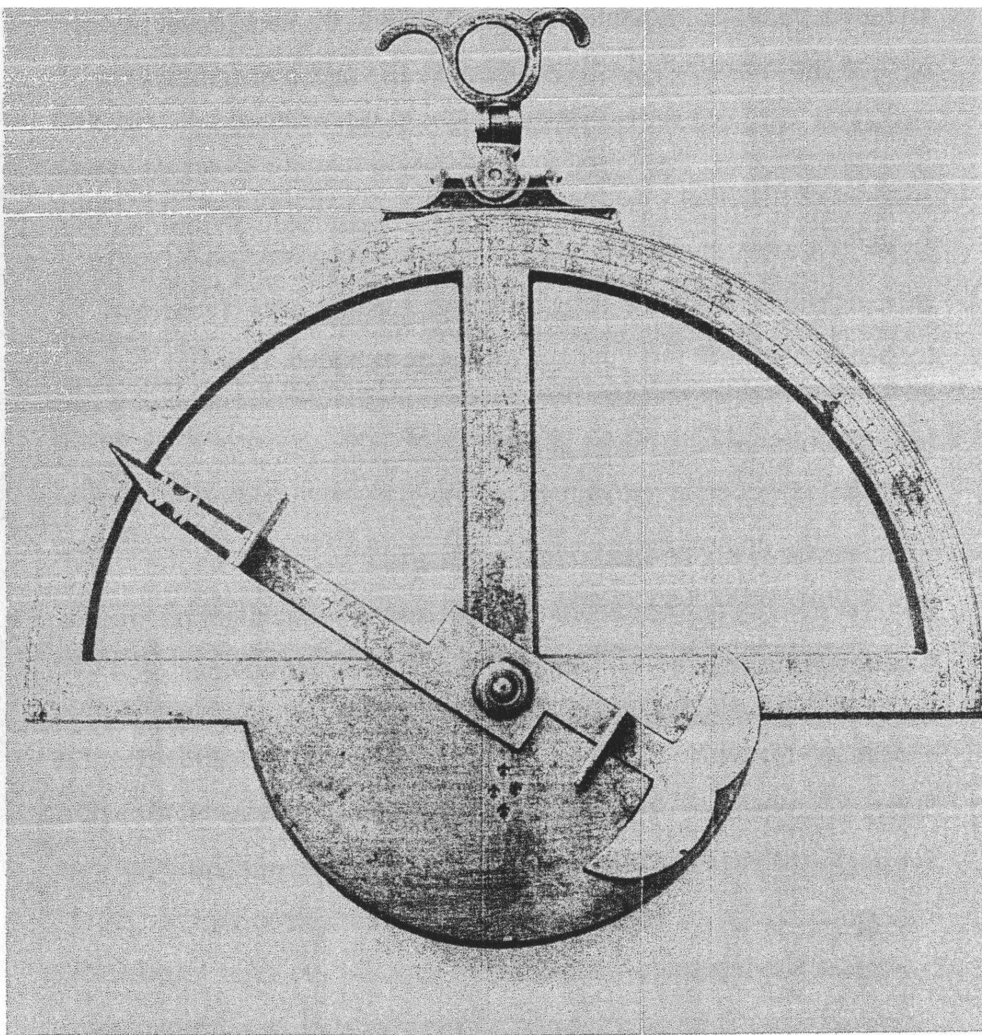
Marineastrolab 1600, støbt i messing, med dobbelt gradinddeling. Højdemålingsinstrument af sjælden type. [Diam. 24 cm].
